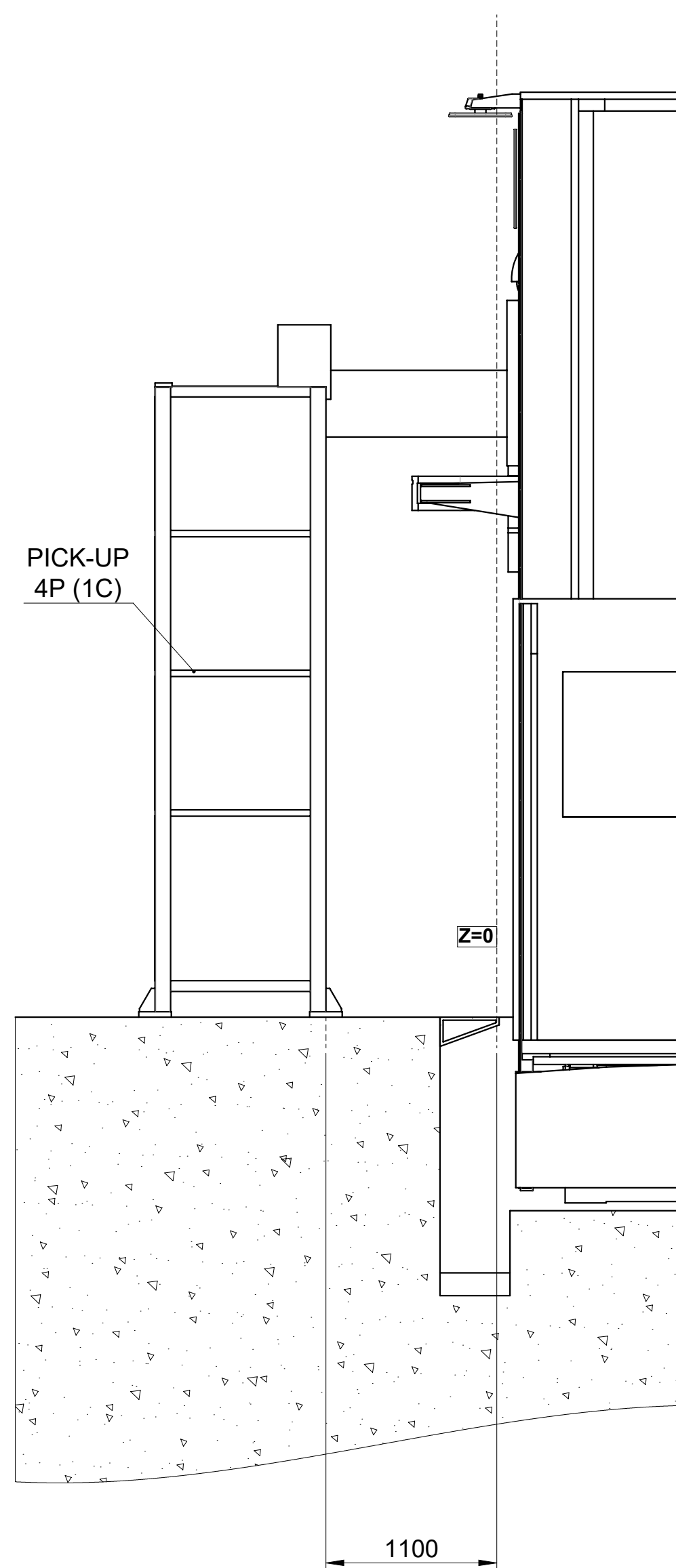
A-A 270°
